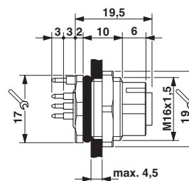
Rysunek wymiarowy
