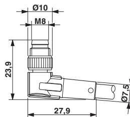
Rysunek wymiarowy
