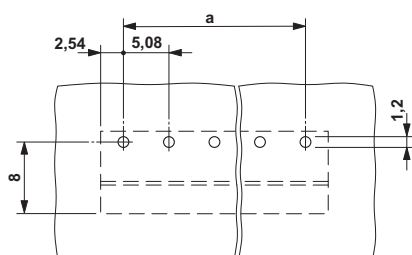
Szablon wierceń
