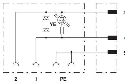
Przyporządkowanie styków wtyków M12 i styków wtyku zaworowego
