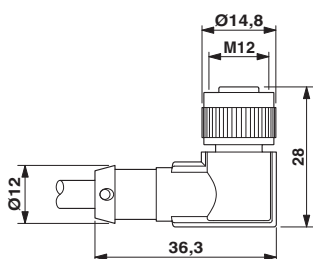
Rysunek wymiarowy
