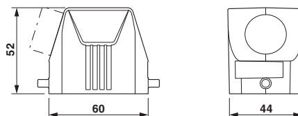
Rysunek wymiarowy
