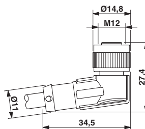
Rysunek wymiarowy
