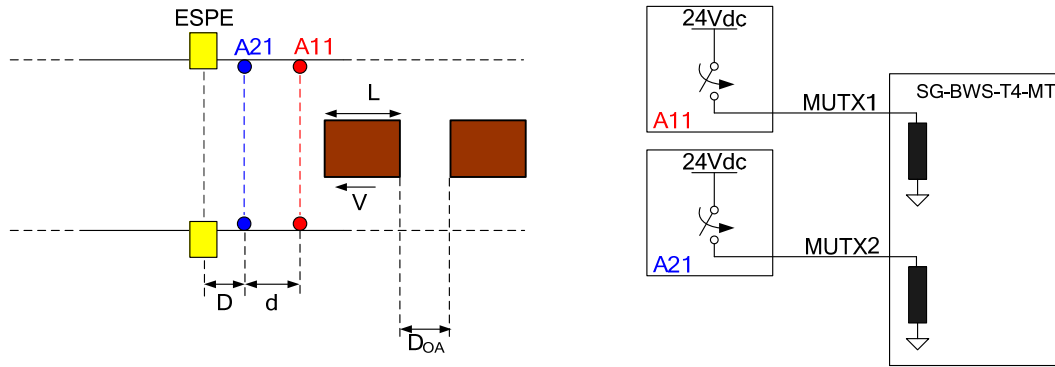
Fig. 32 connessione muting L
