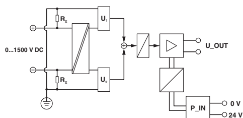
Schemat blokowy
