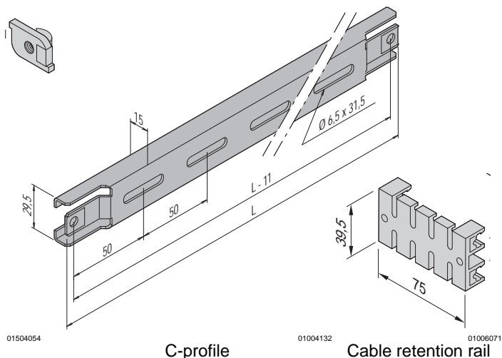
Slide nut
